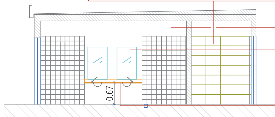
CORTE B'-B' BAÑO CHICAS
