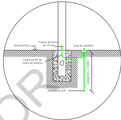
DETALLE PUESTA A TIERRA
