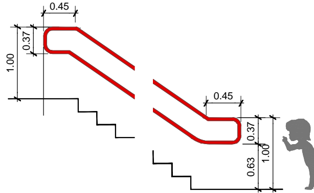
VISTA esc.: 1.50
