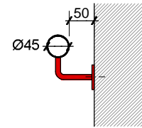
CORTE esc.: 1.10
